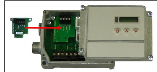
Installation of the USB interface board/ Einbau der USB-Interface-Platine
