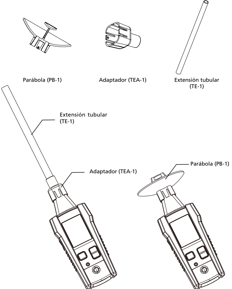
Figura 3.4: Accesorios ULD-400
