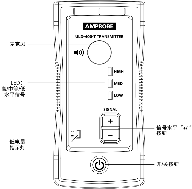
图3.3: ULD-400-T发送器
