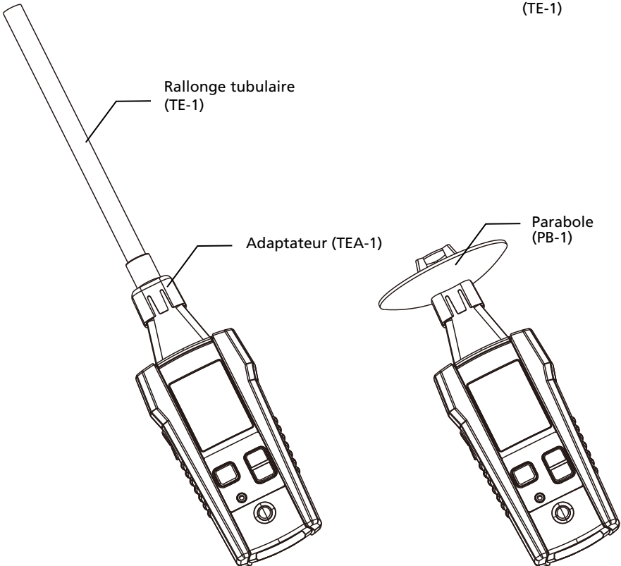
Figure 3.4 : Accessoires du ULD-400
