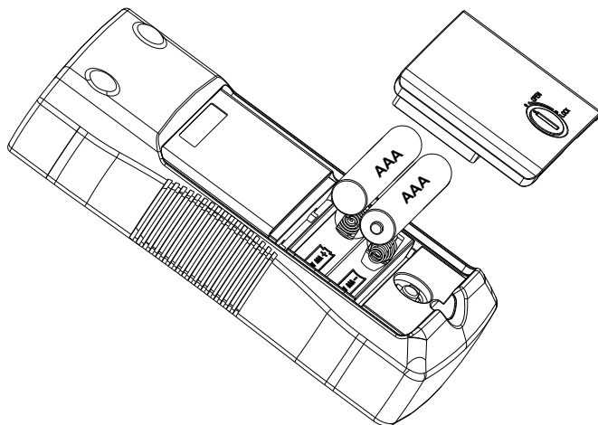
Figura 5.2: Reemplazo de las pilas del Transmisor
