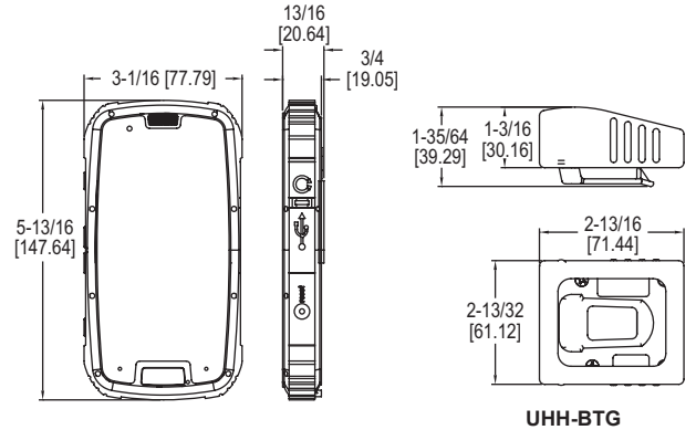
UHH2 Base Unit
