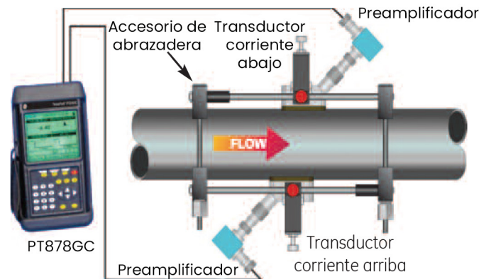
Configuración típica de caudalímetro para caudal de gas con abrazadera portátil
