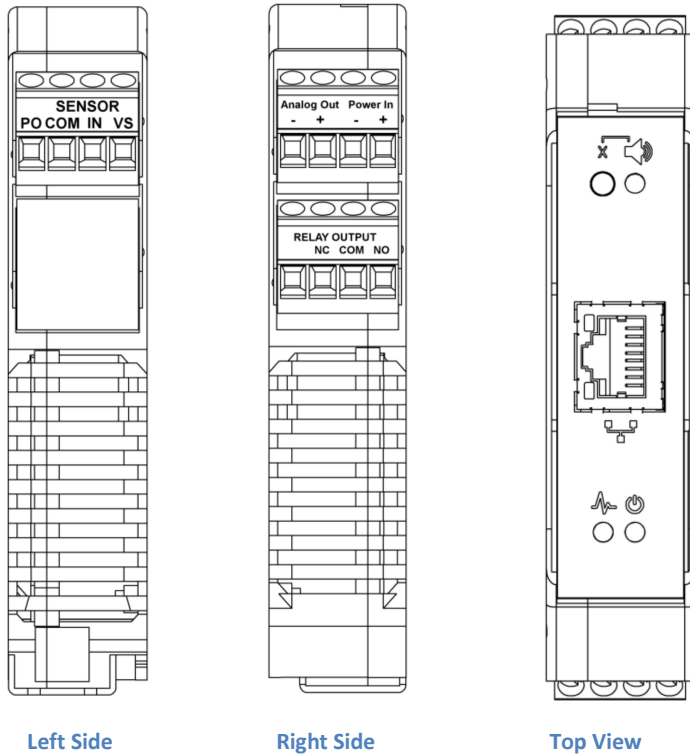
Fig 2.1 – F2A3X Module
