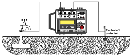
'Dead' earth testing
