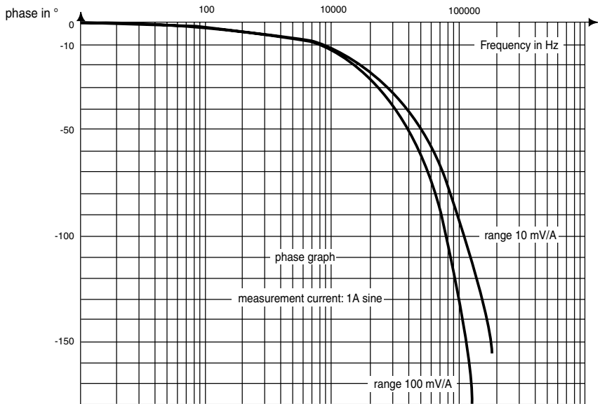
Phase Shift
